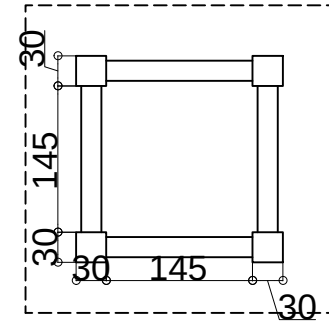
PLAN DE POUTRE
