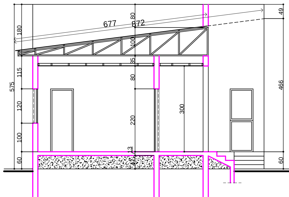
Coupe AA
