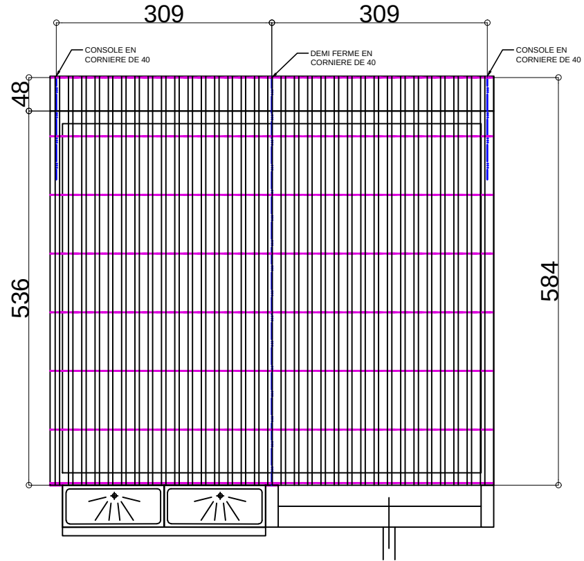
PLAN DE TOITURE
