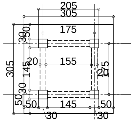
PLAN DE FONDATION
